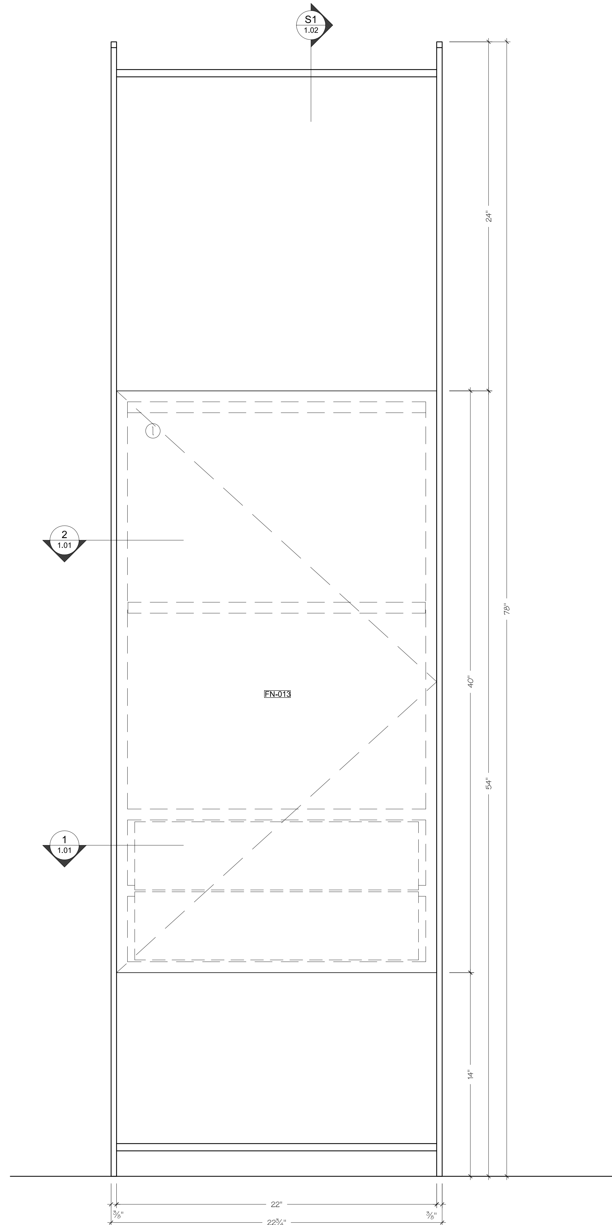
A ELEVATION SCALE: 3" = 1'- 0" LOCKERS
