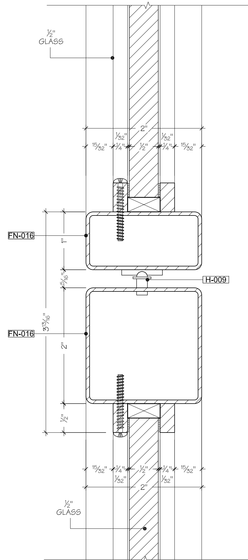
D2 DETAIL SCALE: FULL DOOR D01 ENTRY
