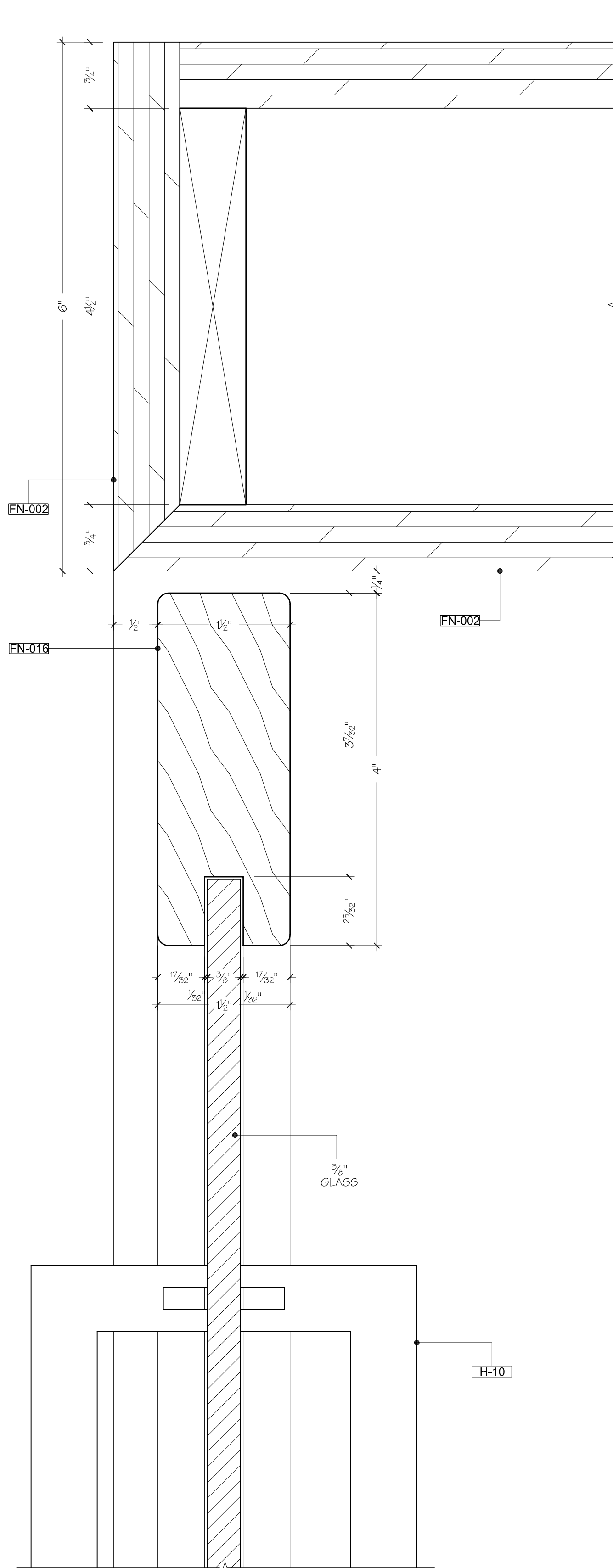
D1 DETAIL SCALE: FULL PHONE BOOTH
