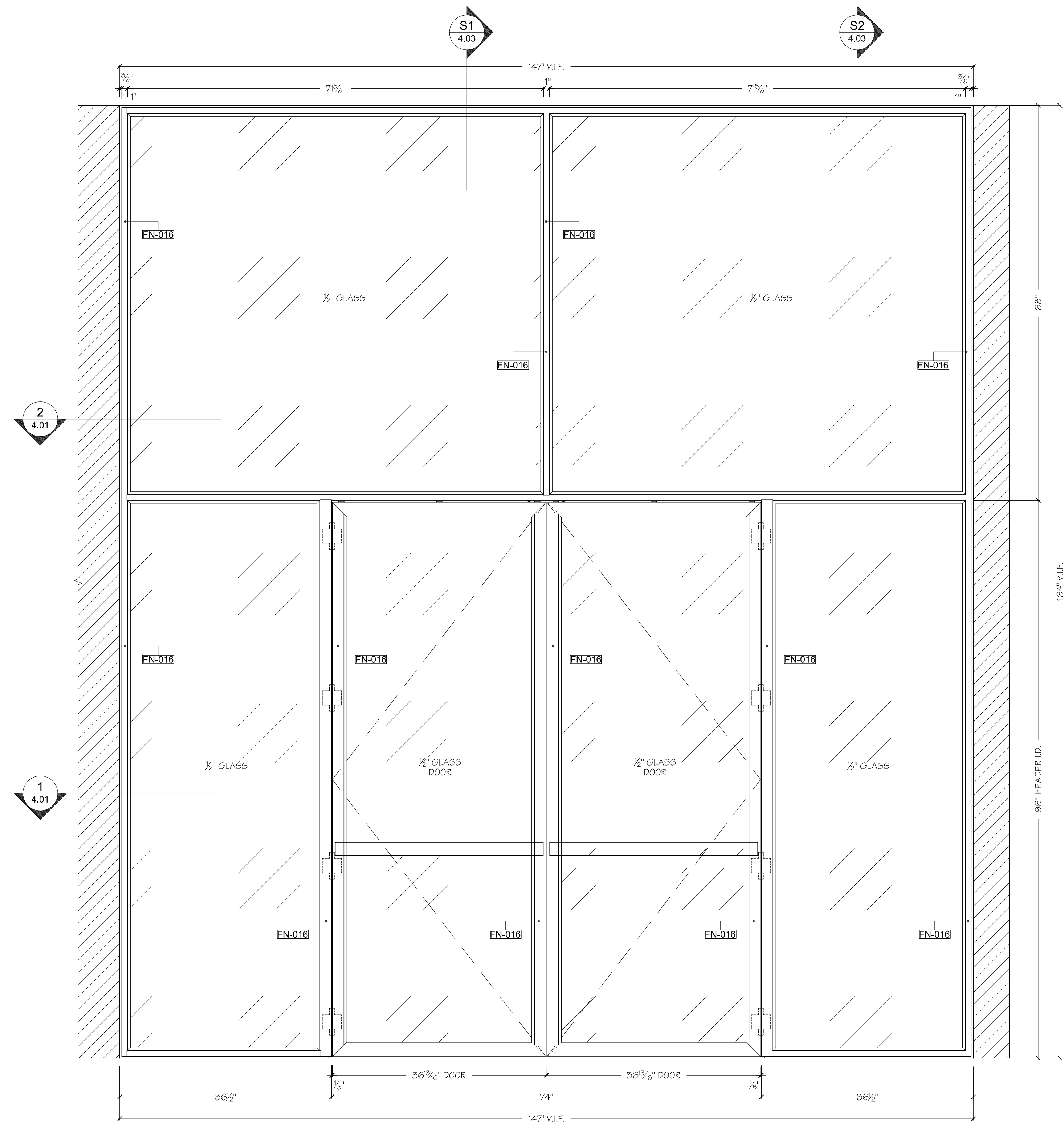
A ELEVATION SCALE: 1" = 1'- 0" DOOR D01 ENTRY
