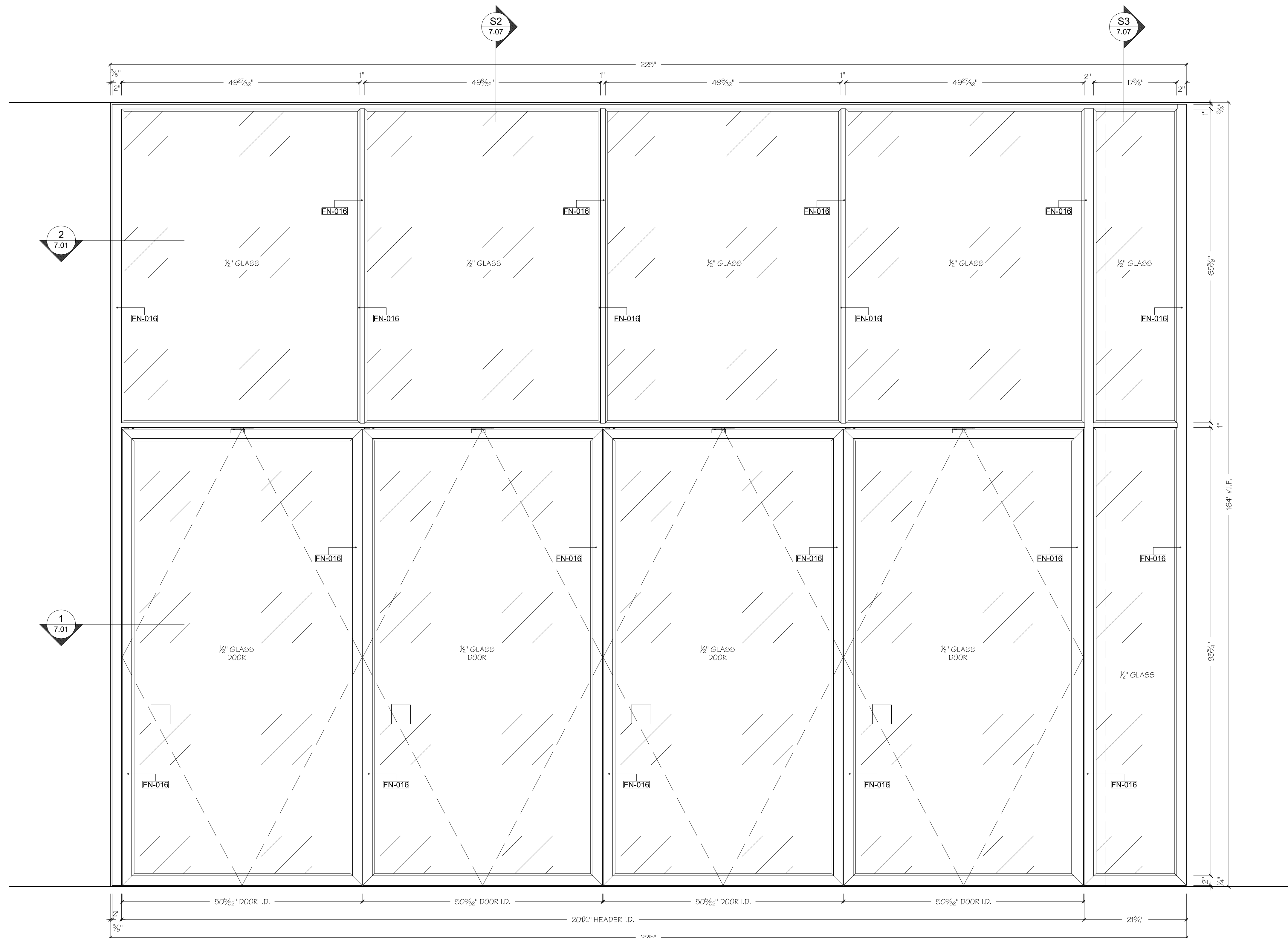
B ELEVATION SCALE: 1" = 1'- 0" PIVOT DOORS
