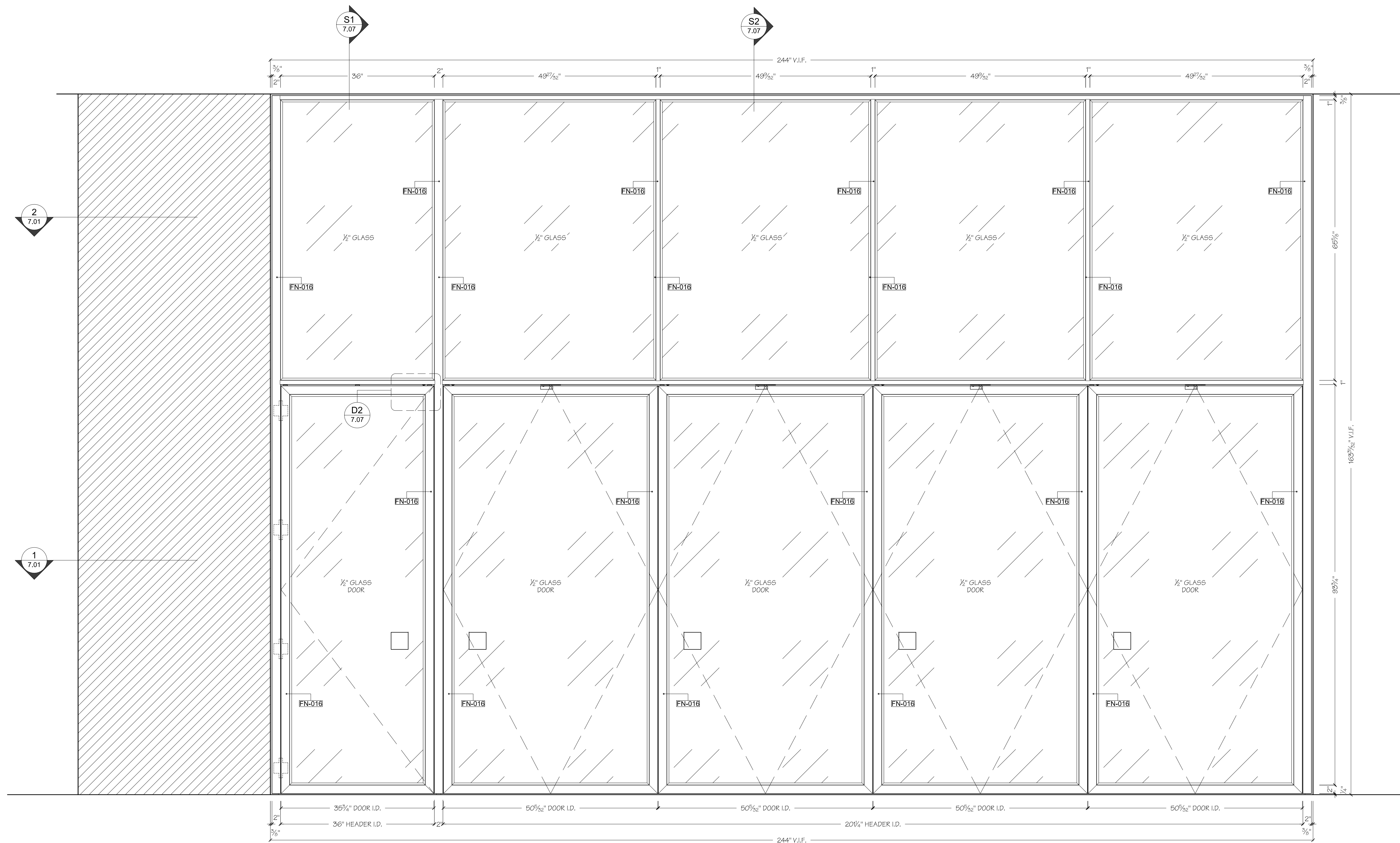
A ELEVATION SCALE: 1" = 1'-0" PIVOT DOORS
