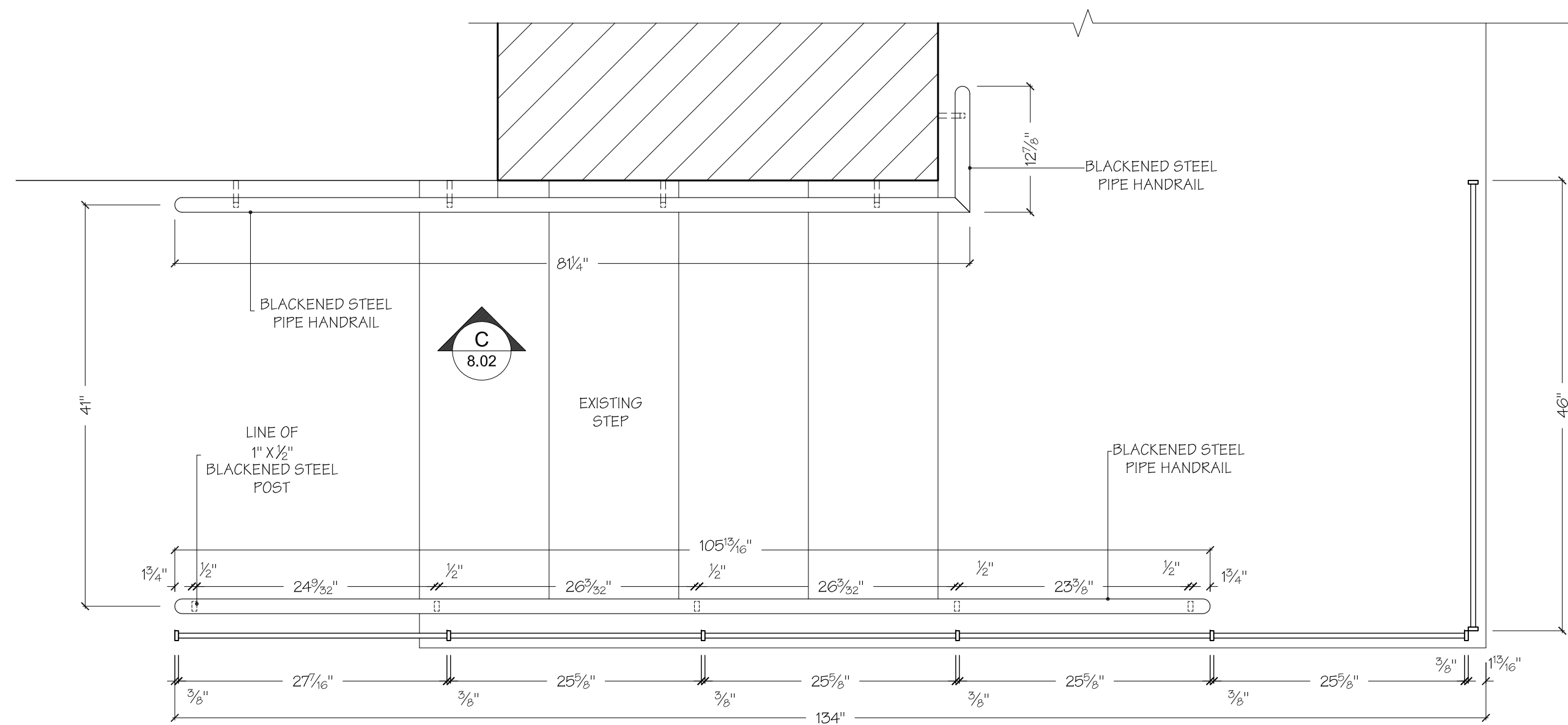
2 PLAN SCALE: 1" = 1'- 0" RAILING
