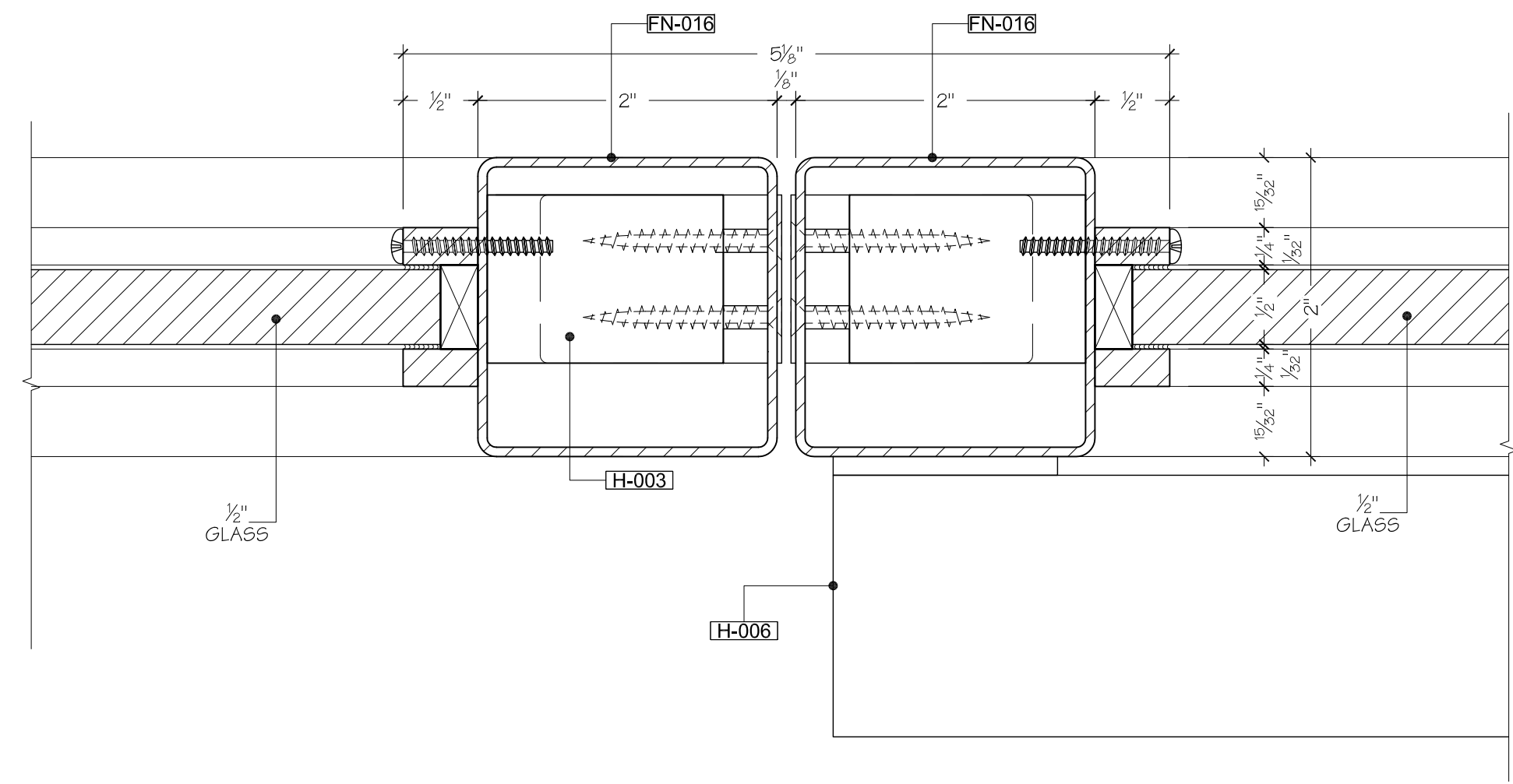
D1 DETAIL SCALE: FULL DOOR D01 ENTRY
