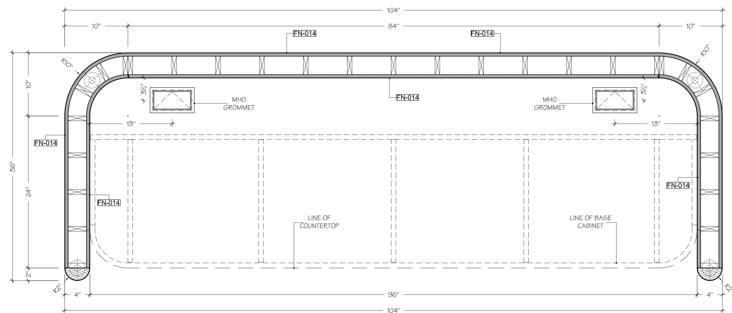
1 PLAN SCALE: 1-1/2" = 1'- 0" RECEPTION
