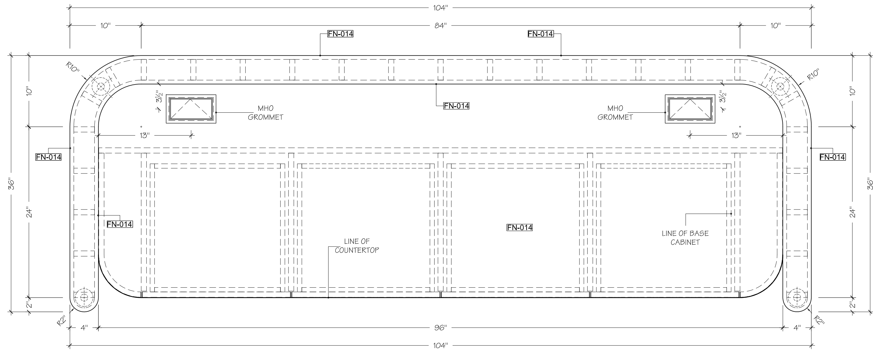
3 PLAN SCALE: 1-1/2" = 1'- 0" RECEPTION
