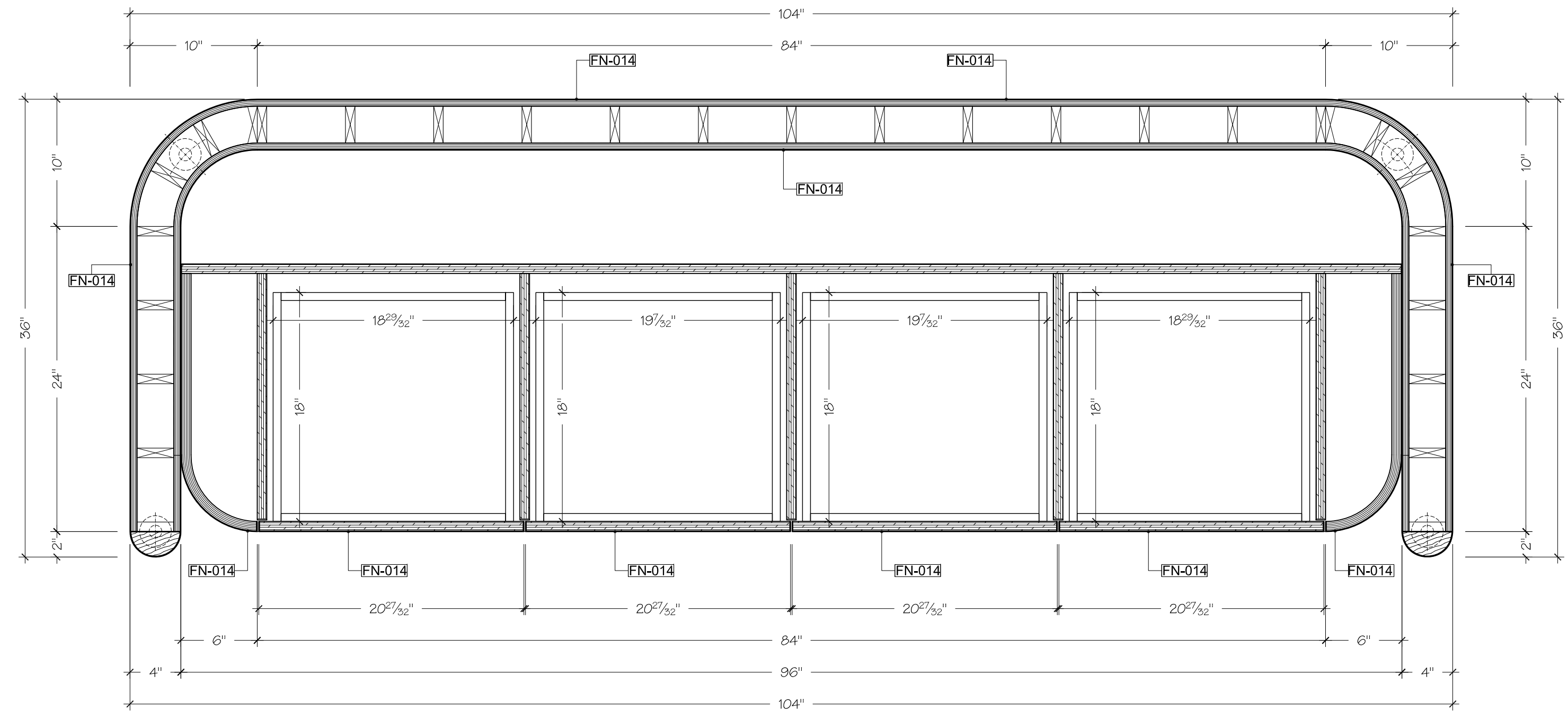
2 PLAN SCALE: 1-1/2" = 1'- 0" RECEPTION
