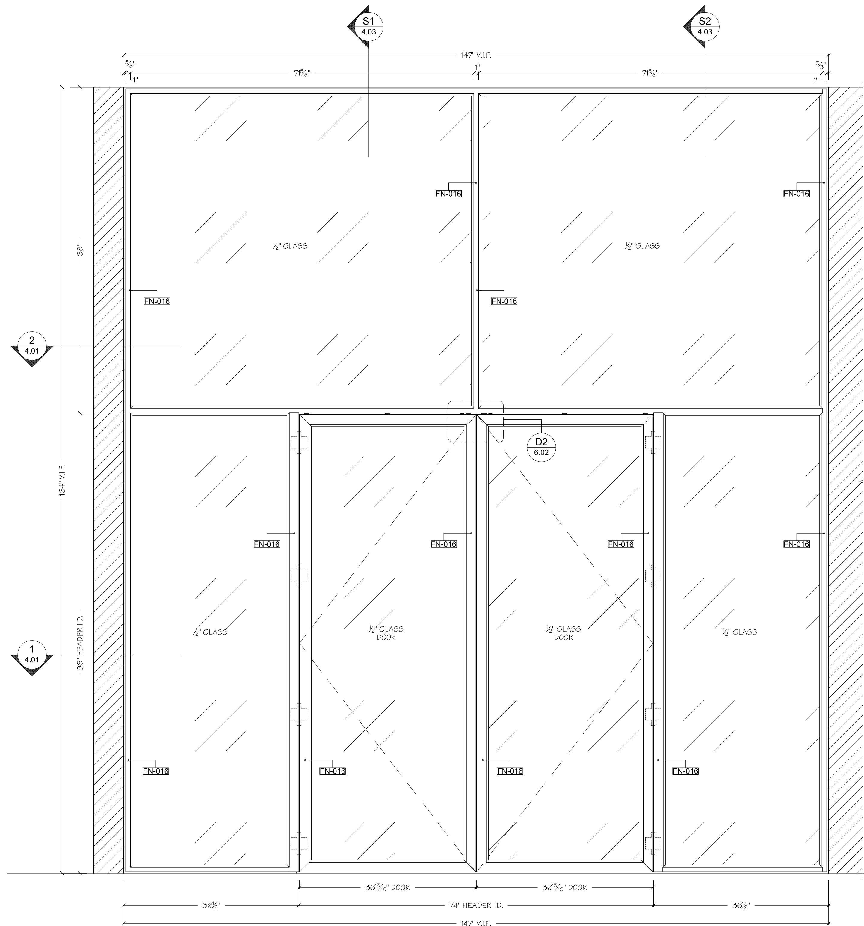
B ELEVATION SCALE: 1" = 1'- 0" DOOR D01 ENTRY
