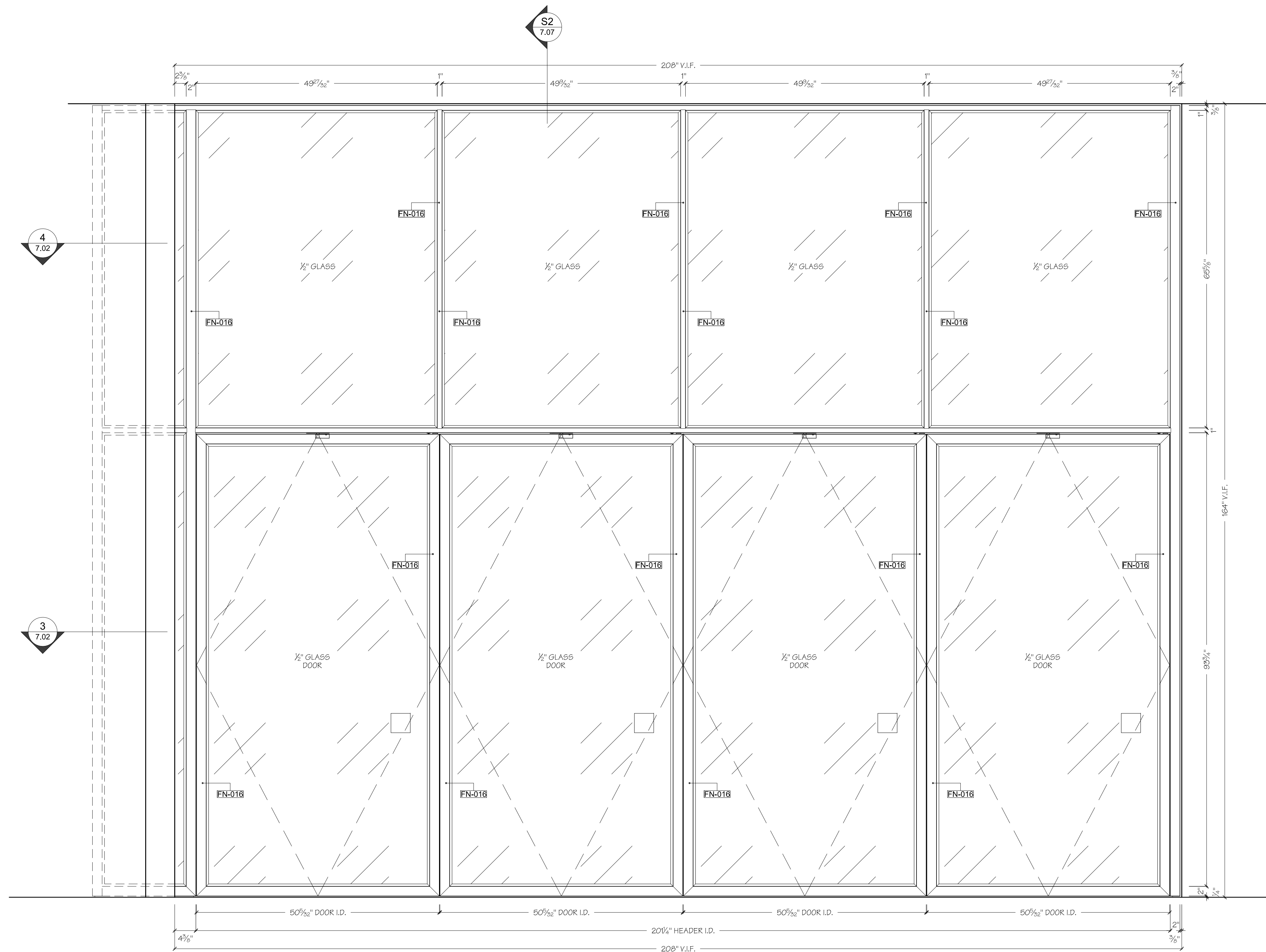
C ELEVATION SCALE: 1" = 1'-0" PIVOT DOORS
