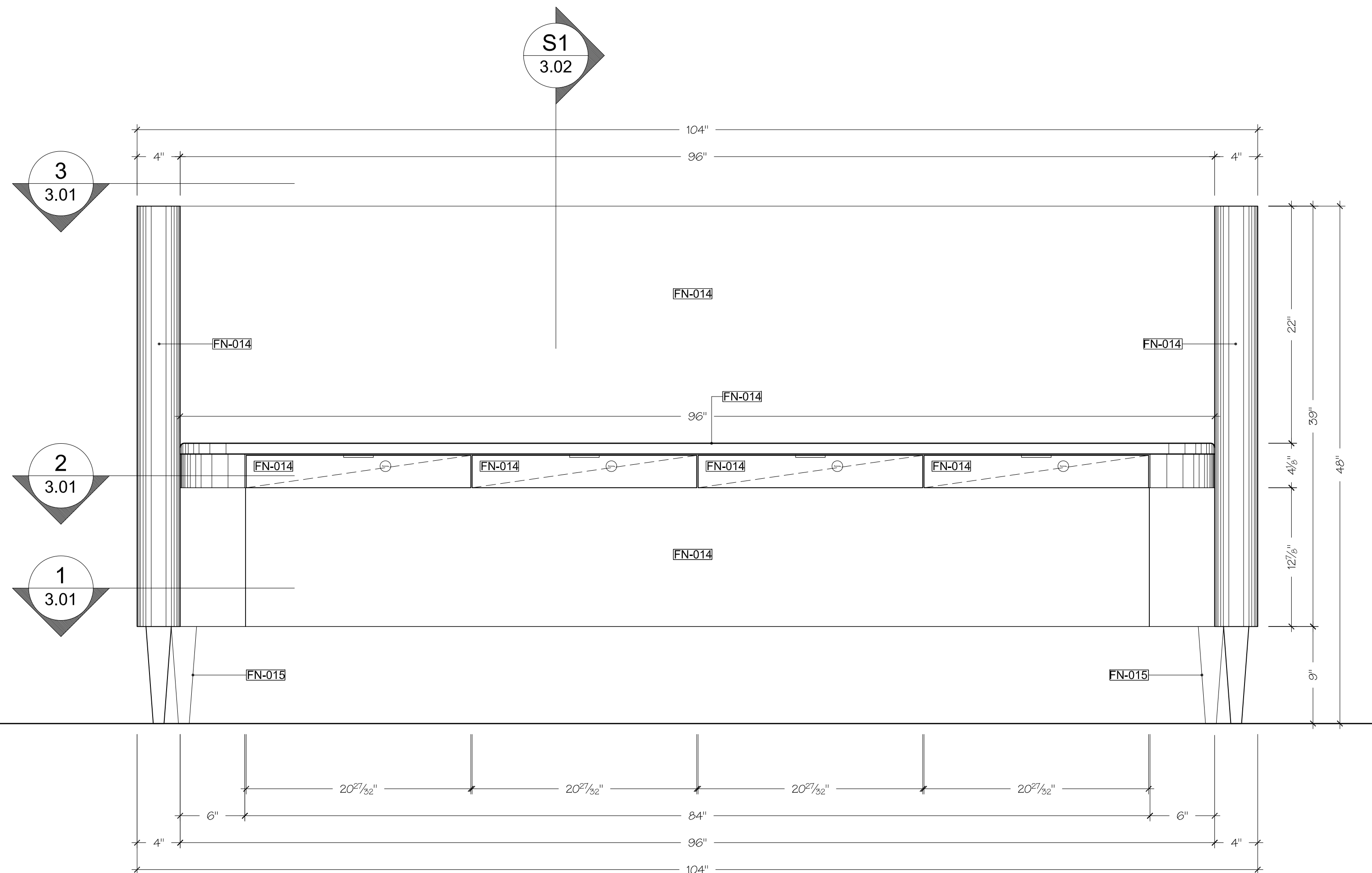
A ELEVATION SCALE: 1-1/2" = 1'- 0" RECEPTION
